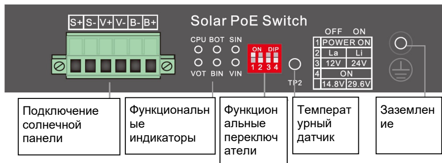
Рисунок 3. Задняя панель.
