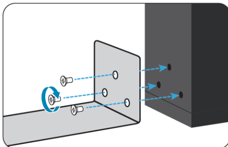
Рисунок 2 – крепление кронштейнов к корпусу
