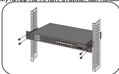
Рисунок 4 – крепление коммутатора на RACK-стойке
