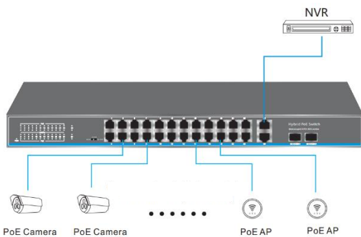
Рисунок 5 – схема подключения устройств к коммутатору
