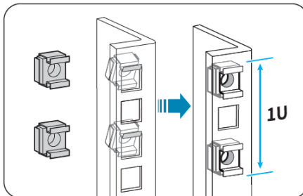
Рисунок 3 – установка «плавающих» гаек
