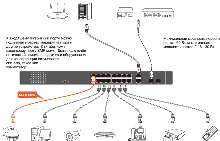
Рисунок 6 – схема подключения устройств к коммутатору
