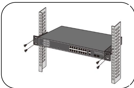
Рисунок 4 – крепление коммутатора на RACK-стойке
