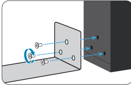
Рисунок 2 – крепление кронштейнов к корпусу
