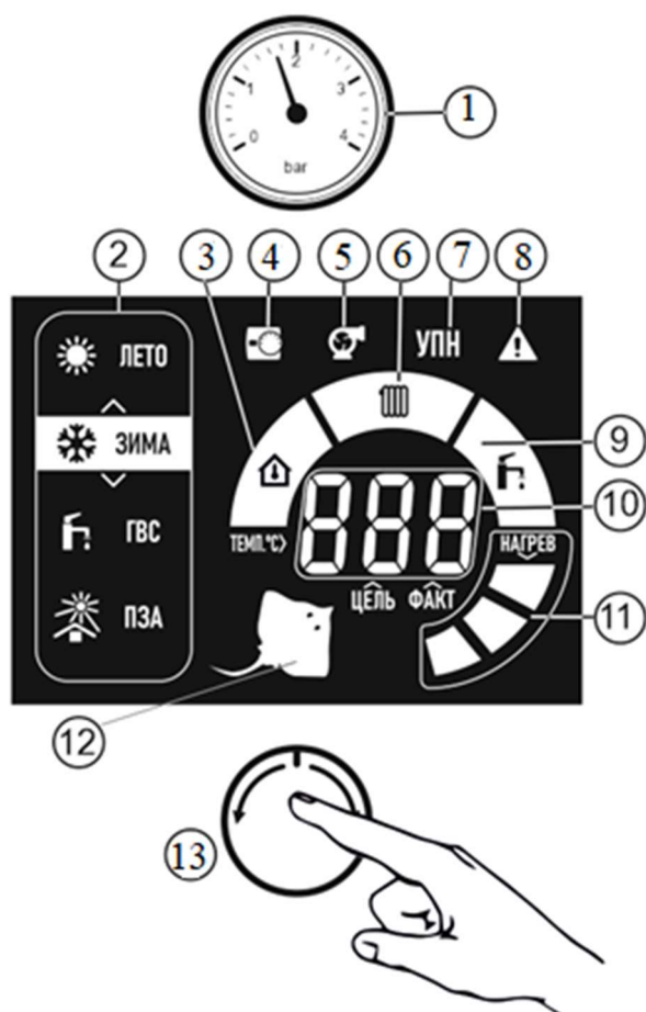
Рисунок 2 - Органы индикации и управления
