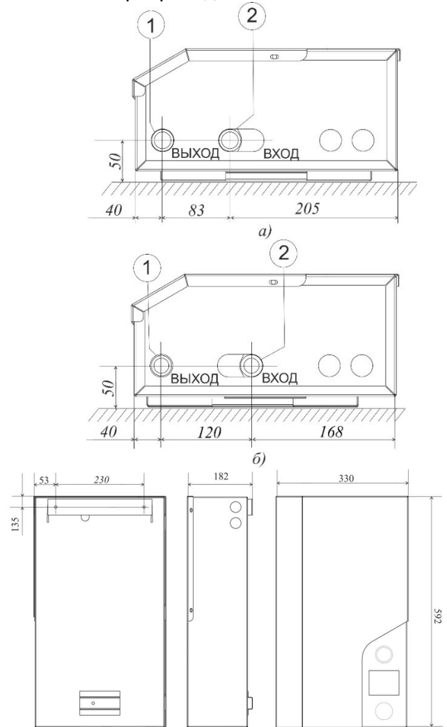
Рисунок 3 - Монтажные размеры электрокотла:
