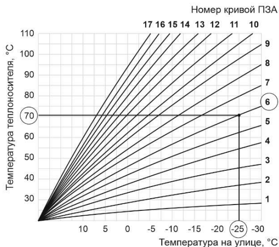
Рисунок 8 - Кривые зависимости температуры теплоносителя от температуры на улице
