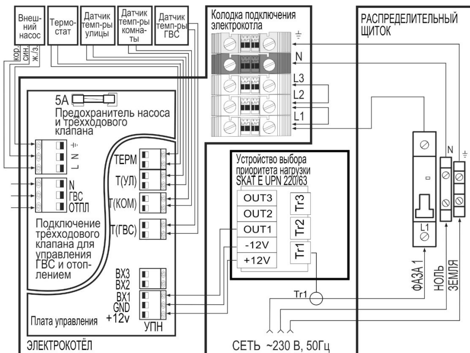
Рисунок 6 - Схема подключения электрокотла к сети ~230 В
