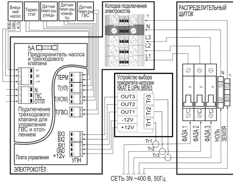
Рисунок 5 - Схема подключения электрокотла к сети 3N ~400 В
