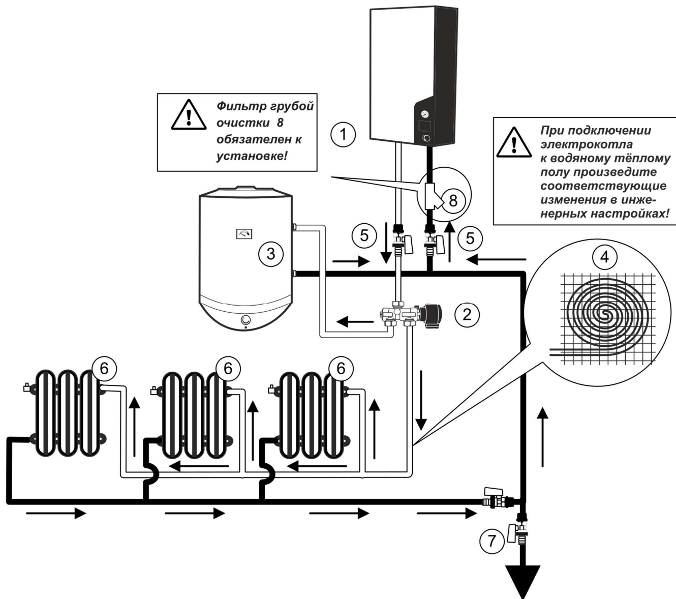
Рисунок 4 - Примерная схема устройства отопительной системы
