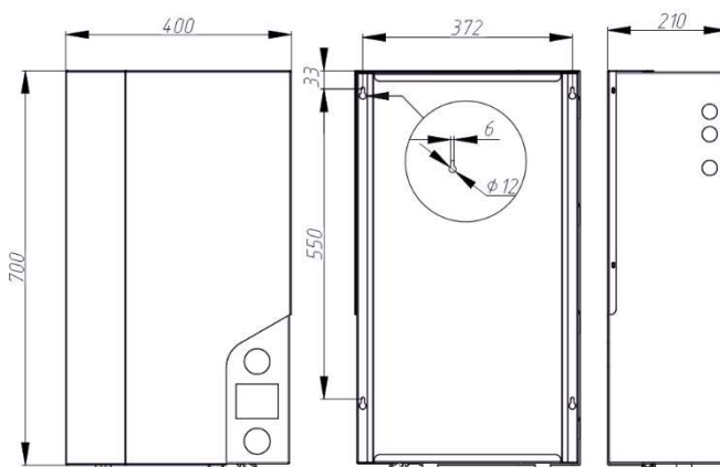
Рисунок 3 - Монтажные размеры электрокотла.
