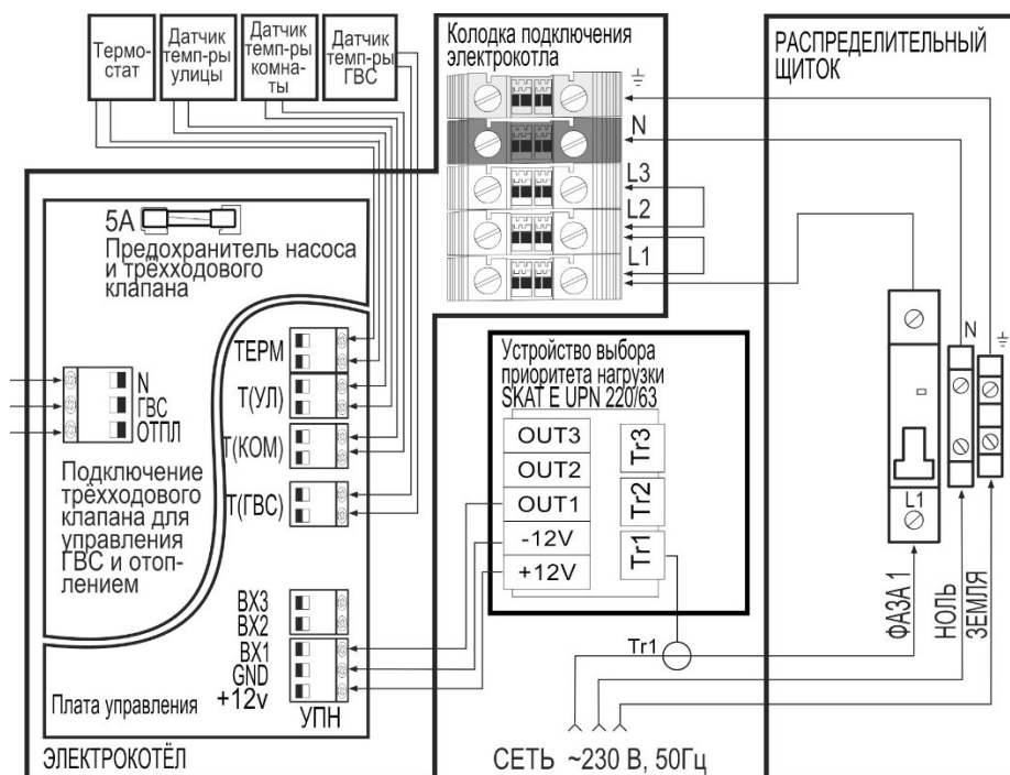
Рисунок 6 - Схема подключения электрокотла к сети ~230 В
