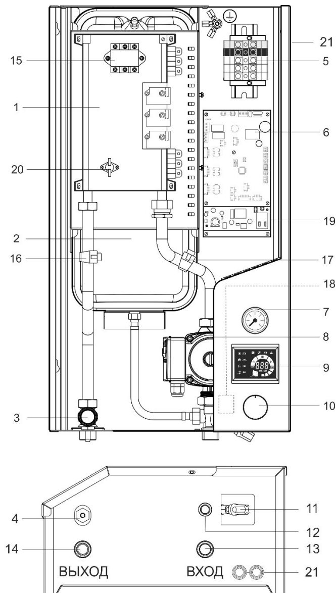
Рисунок 1 - Схема внутреннего устройства электрокотла
