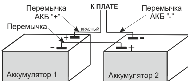
Рисунок 3 – Подключение АКБ
