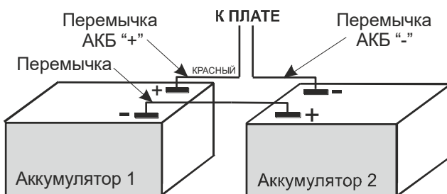
Рисунок 3 – подключение АКБ
