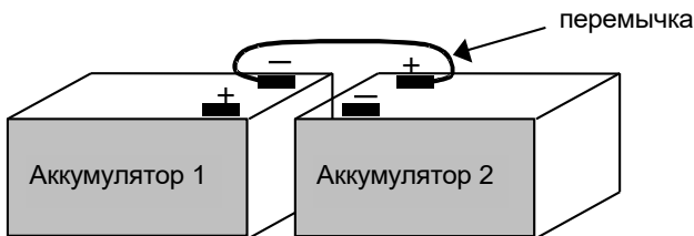
Рисунок 2 – Схема последовательного соединения двух аккумуляторов
