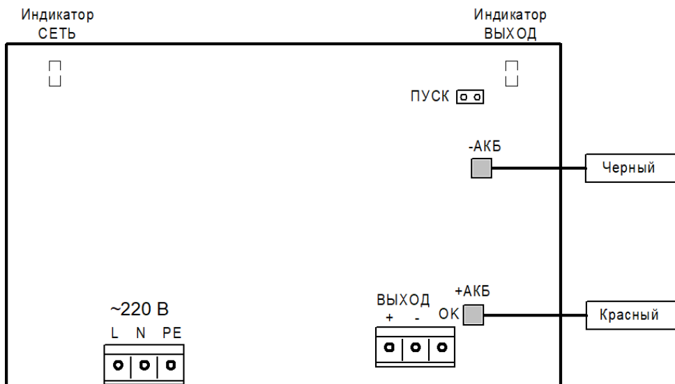
Рисунок 1 - Вид изделия с открытой крышкой (схема подключения)
