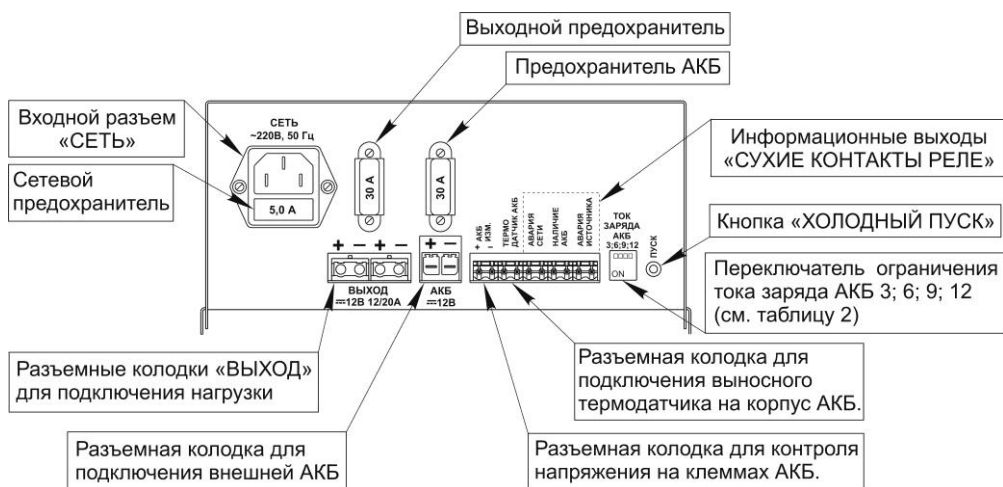
Рисунок 2 – Задняя панель изделия
