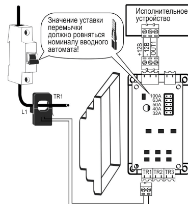
Рисунок 4 – Схема однофазного подключения
