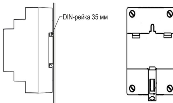
Рисунок 1 – Крепление изделия
