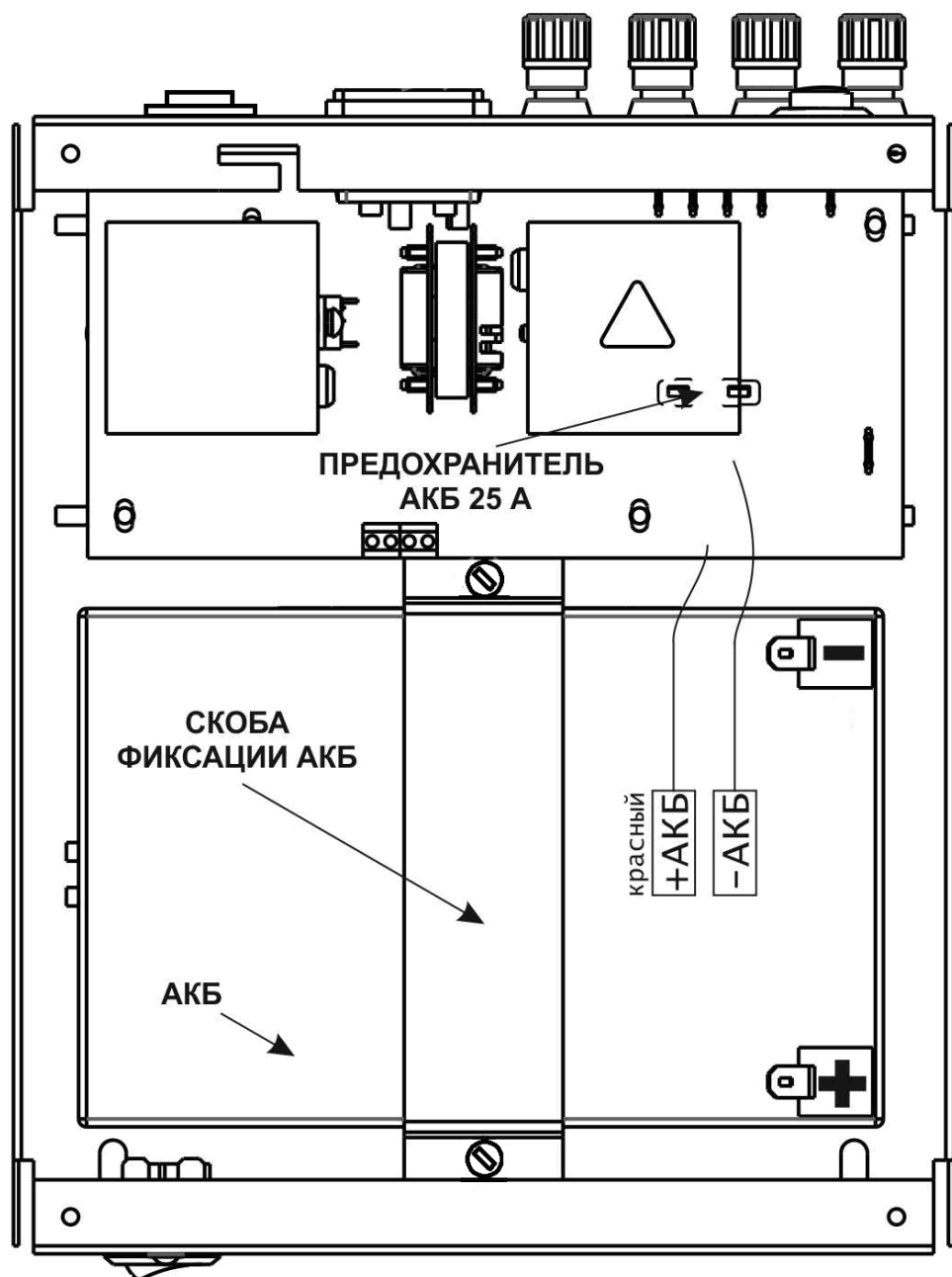
Рис.3 Расположение коммутационных элементов ВОЛНА ББП – 3/20 при снятой крышке корпуса
