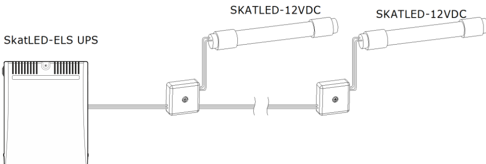
Рисунок 3 – Схема подключения светильников аварийного освещения
