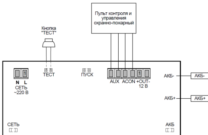
Рисунок 2 – Схема подключения (вид снизу)
