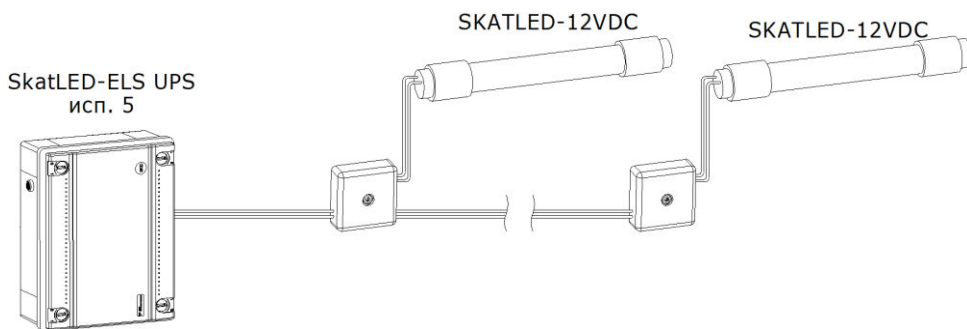
Рисунок 4 – Схема подключения светильников аварийного освещения.
