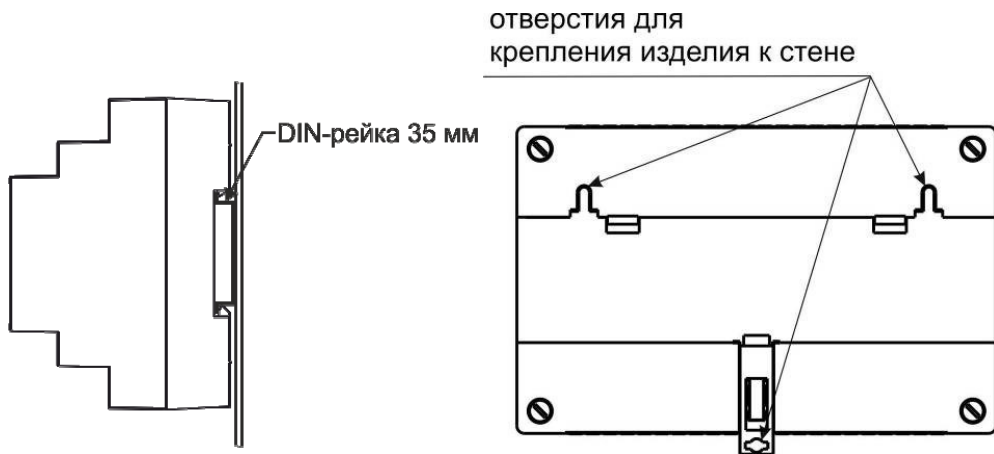
Рисунок 1 - Крепление изделия
