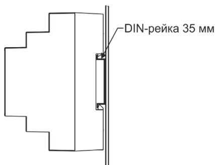
Рисунок 2 – Установка изделия
