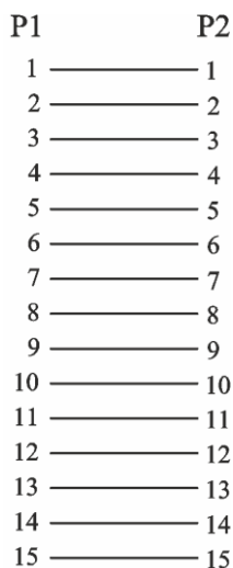
Рисунок 2 — Схема подключения
