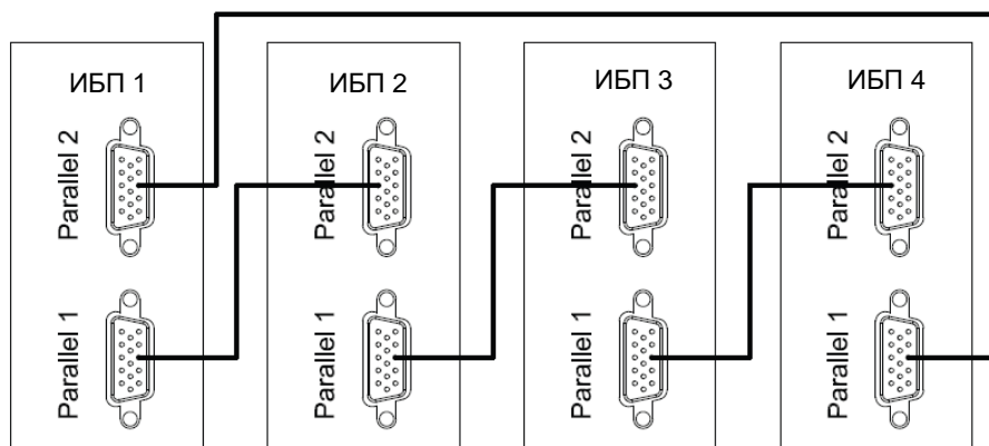
Рисунок 3 – Схема соединения изделий в «кольцо» через параллельные порты
