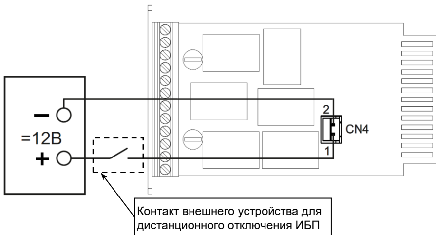
Рисунок 4 — Пример схемы подключения контакта внешнего устройства мониторинга
