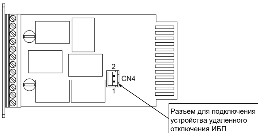
Рисунок 2 — Вид модуля сверху
