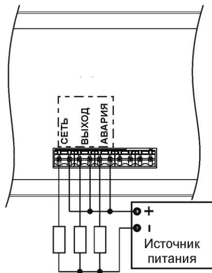
Рисунок 5 – Подключение внешних устройств автоматики
