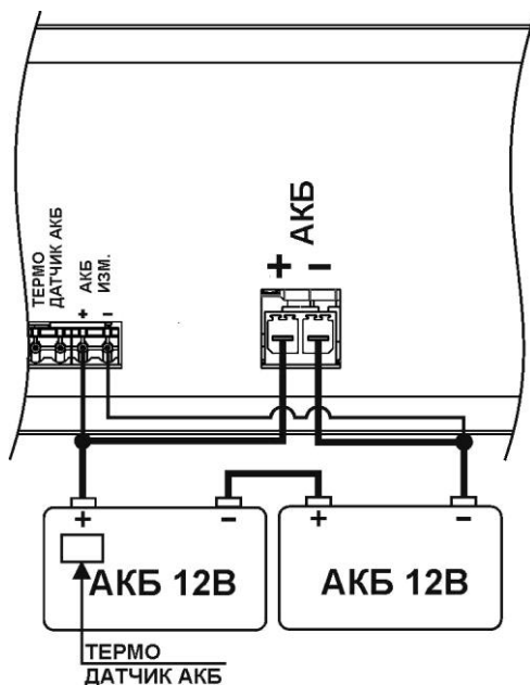
Рисунок 4 – Подключение АКБ и термодатчика АКБ.
