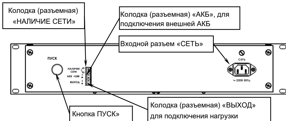
Рисунок 2 – задняя панель изделия
