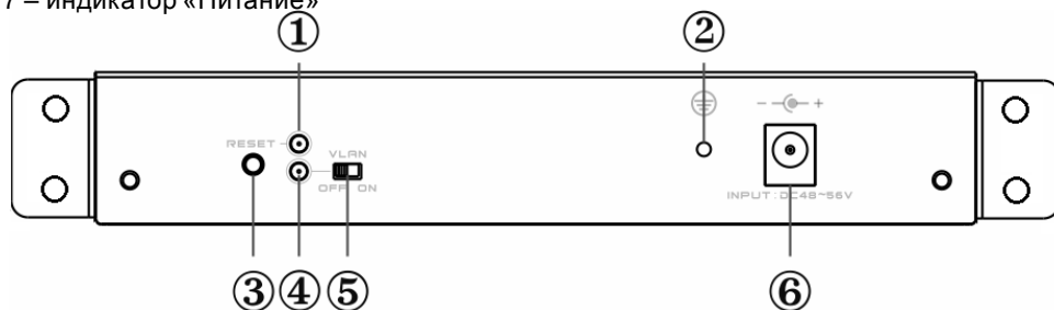
Рисунок 5 – задняя панель коммутатора**
