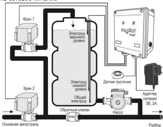
Рис. 3 – Схема подключения
