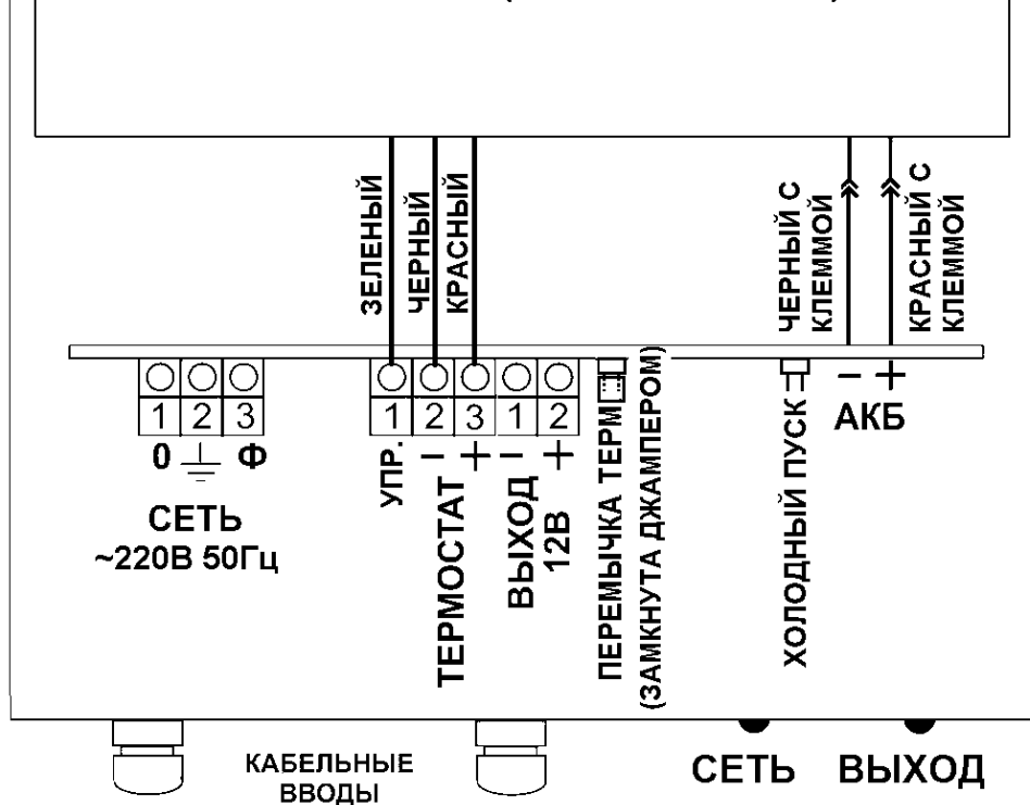
Рисунок 3. Экономичный вариант подключения термостата АКБ к изделию (с отключением термостатирования в режиме «Резерв»)
