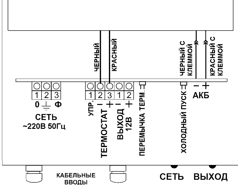
Рисунок 2. Стандартный вариант подключения термостата АКБ к изделию (без отключения термостатирования в режиме «Резерв»)
