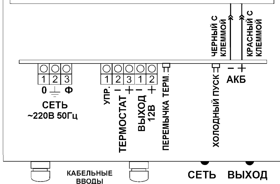
Рисунок 1 - вид изделия с открытой крышкой (схема подключения)
